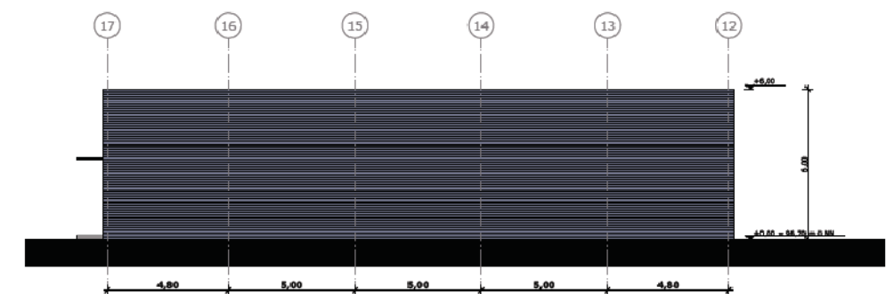
Ansicht Nord-West
