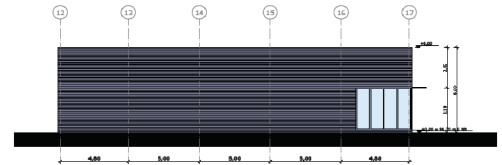
Ansicht Süd-West
