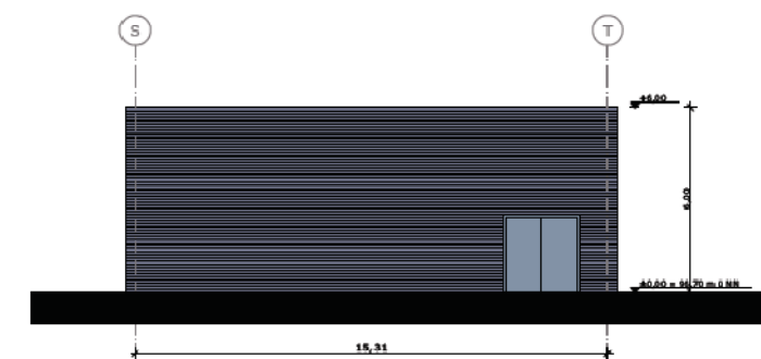
Ansicht Süd-West
