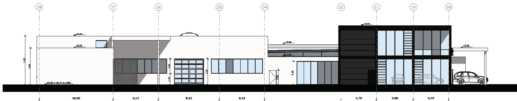
Ansicht Süd-West
