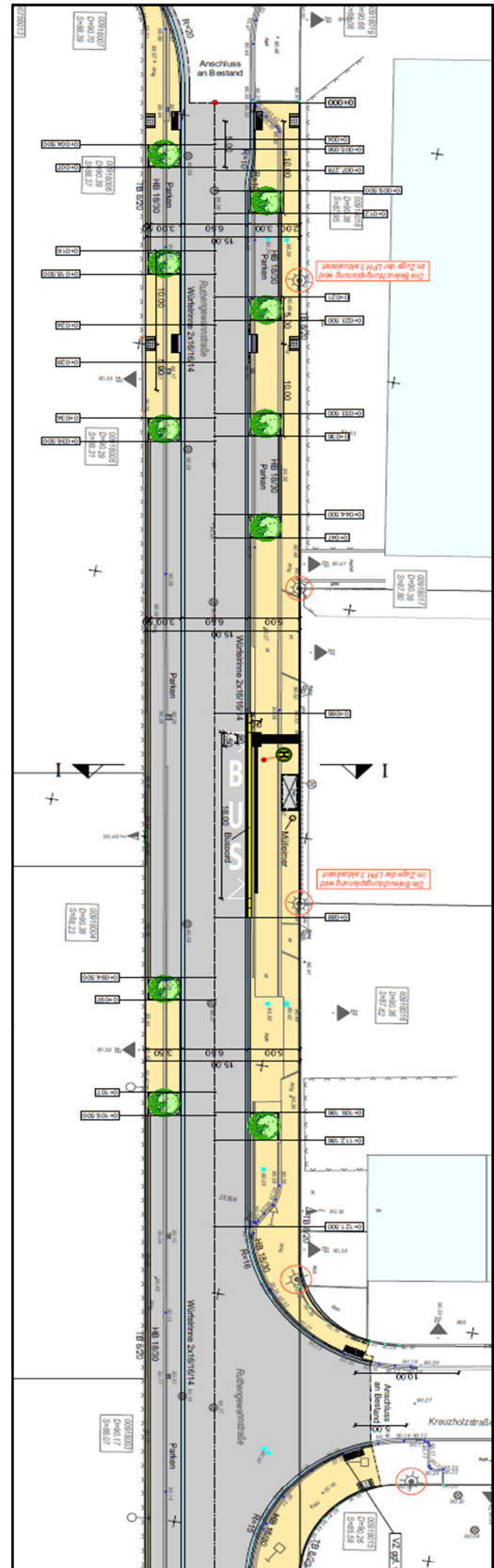
Lageplan Nordteil
