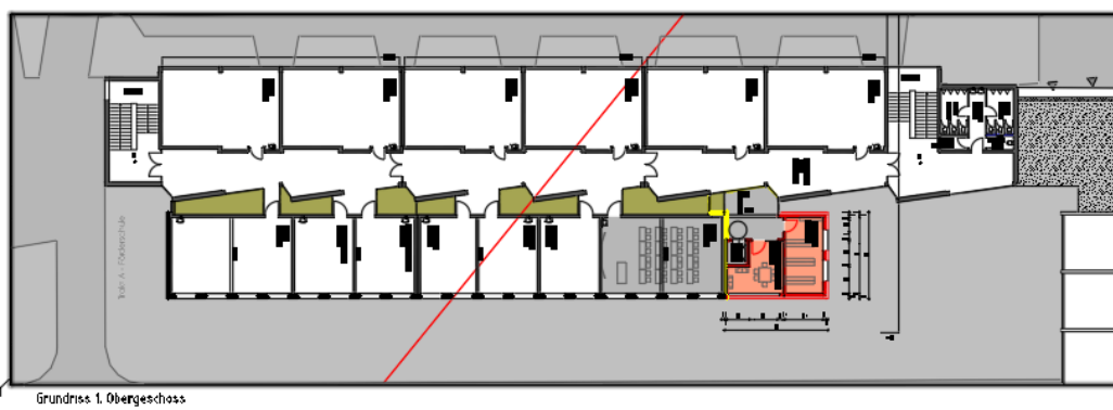
Lupe C Trakt Fördererschule Erdgeschoss, Obergeschoss
