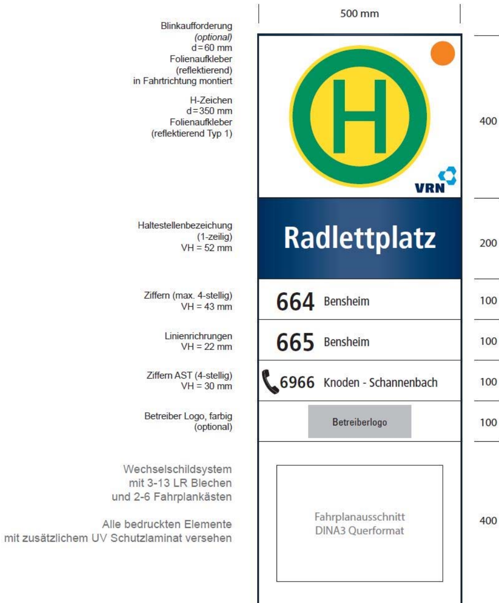
Abbildung 42: Wechselschild mit gewölbter Oberfläche als Stele (höherwertiges System)
