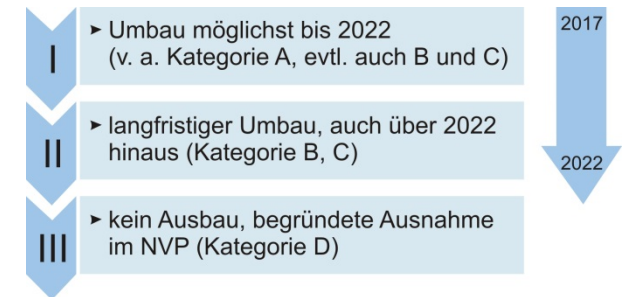
Abbildung 20: Haltestellenpriorisierung
