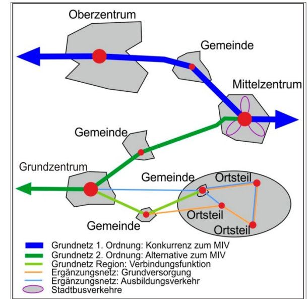
Abbildung 2: Netzhierarchie
