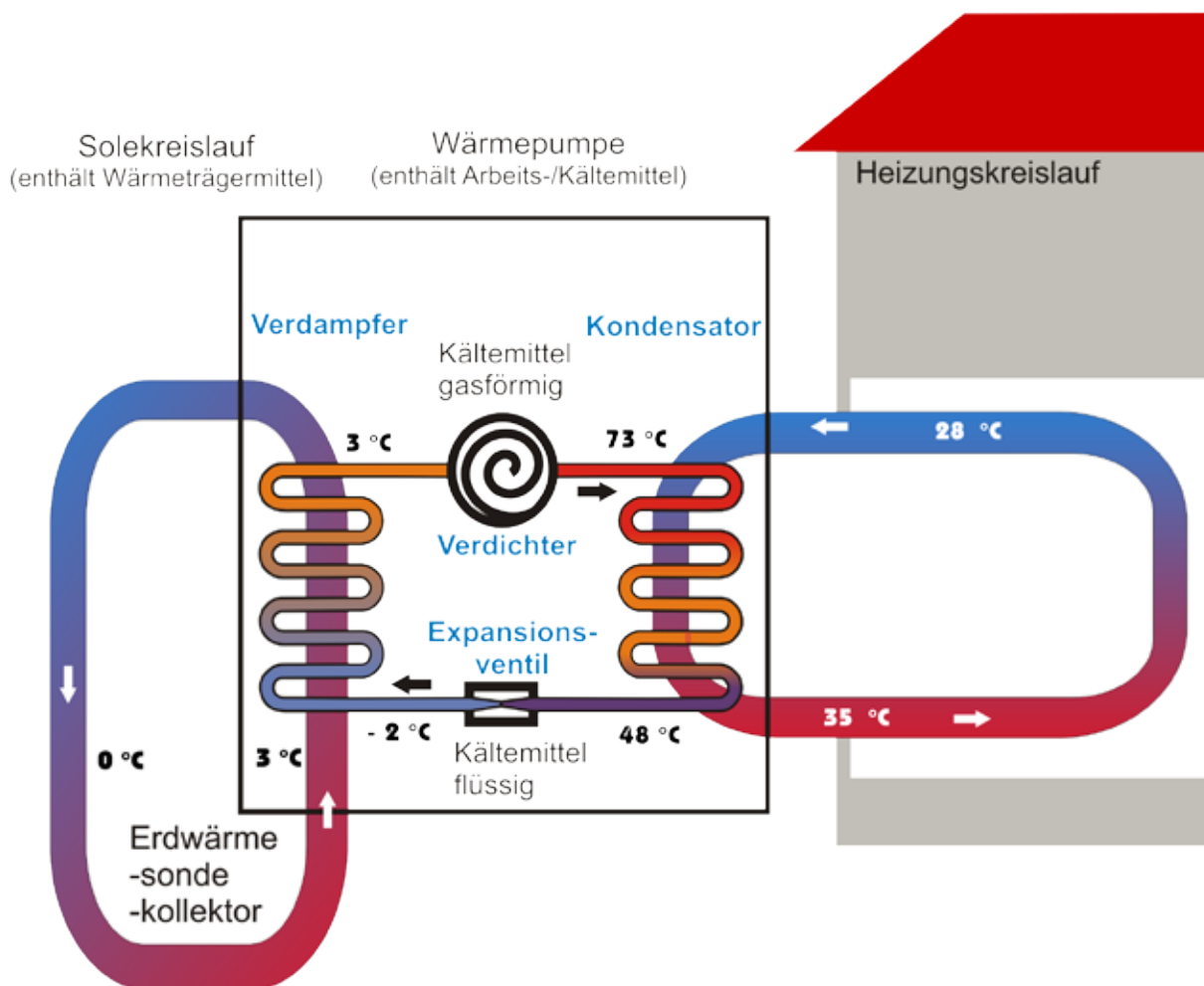
Abb. 3 : Schema zur Erdwärmegewinnung
